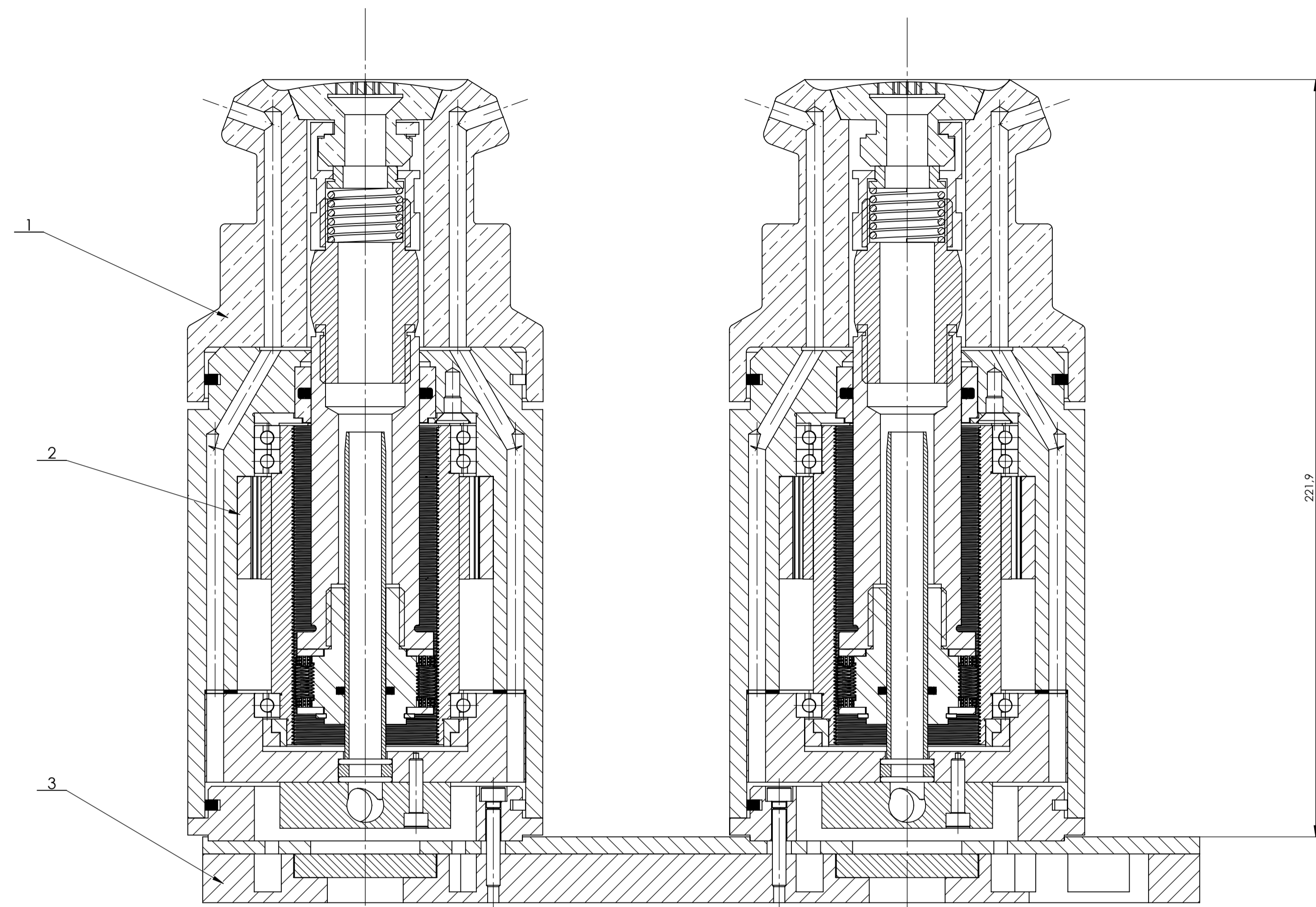
ŘEZ A-A MĚŘÍTKO 1:1
