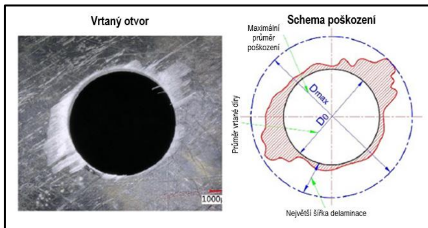
Obrázek 8 – znázornění oblasti poškození delaminací [16]
