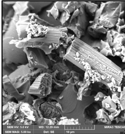
Obrázek 18 – snímek částic uhlíkových vláken v epoxidové pryskyřici vzniklých při vrtání nástrojem SK.
