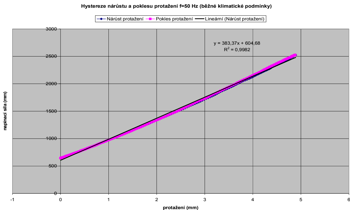
Graf 3 Hystereze při frekvenci protahování 50 Hz
