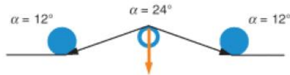
Obr. 3 Použití snímače na rovném úseku nitě s obvyklými úhly opásání dle [14]
