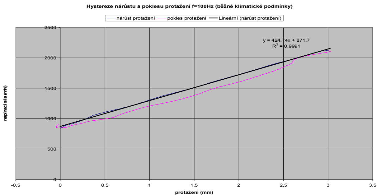
Graf 4 Hystereze při frekvenci protahování 100 Hz
