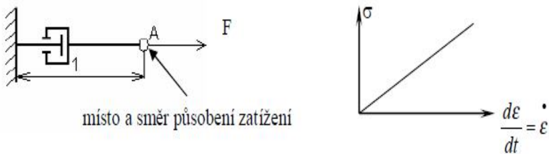
Obr. 22 Model Newtonovské kapaliny a pracovní diagram dle [12]
