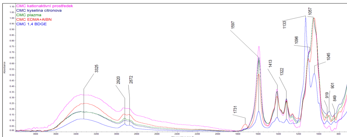
Graf 24 Souhrnné spektrum chemicky a radiačně upravených filmů
