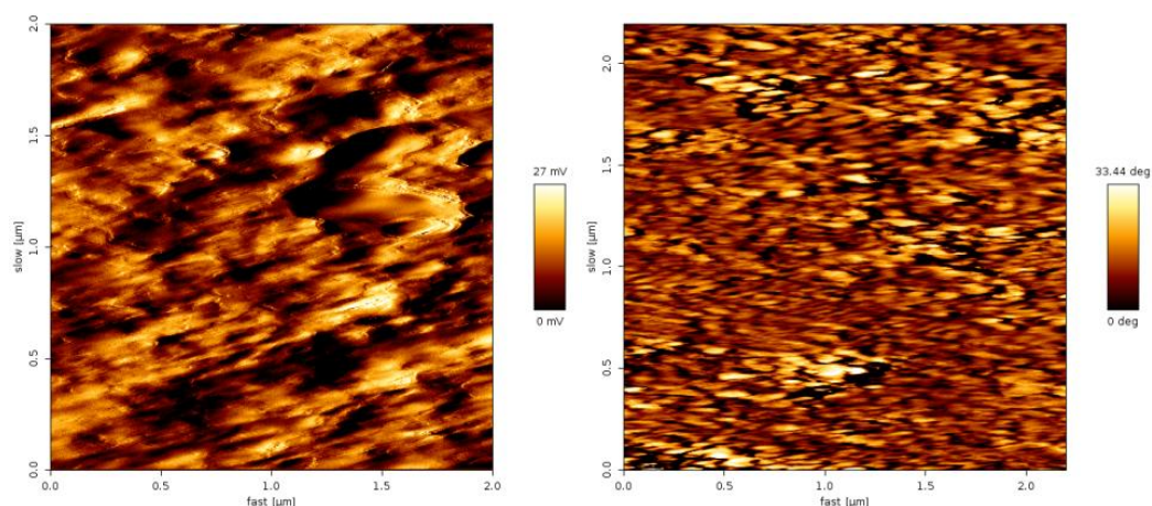
Obr. 41 a) povrchová struktura neoplazmovaného vzorku; b) povrchová struktura neoplazmovaného vzorku
