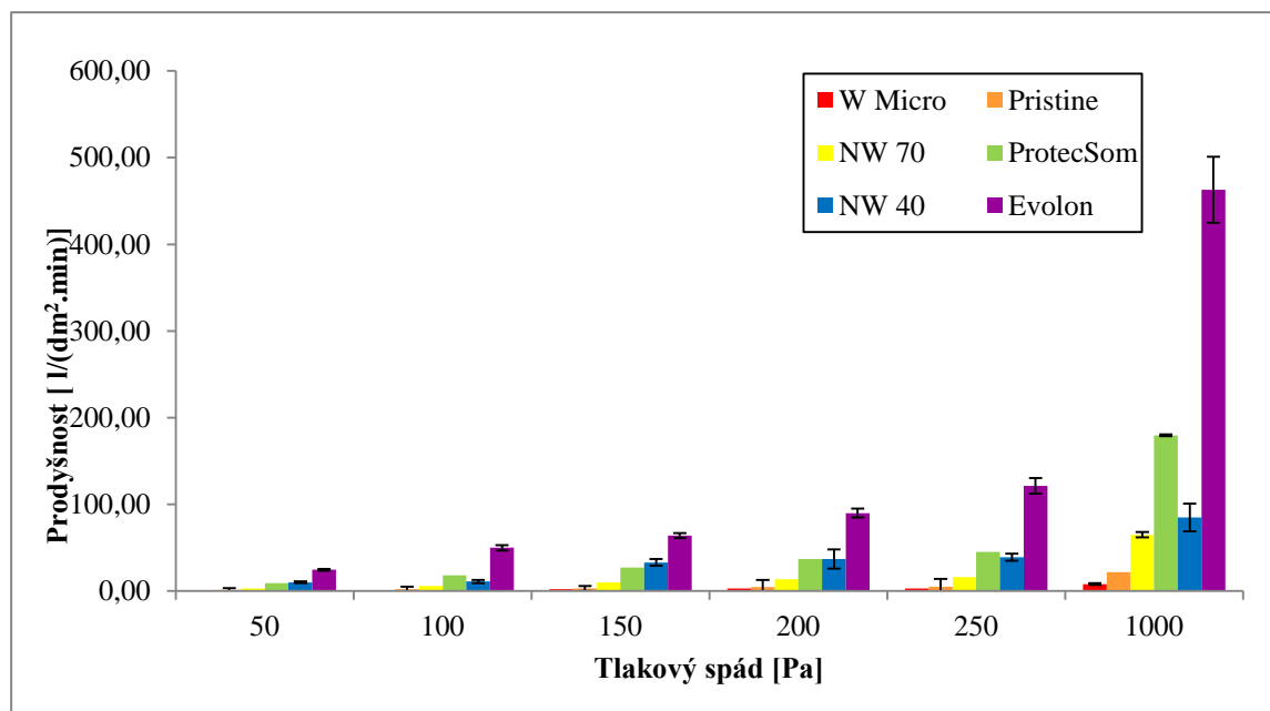
Obr. 19: Průměrné hodnoty prodyšnosti při různých tlakových spádech.
