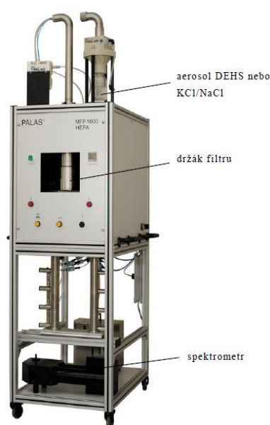
Obr. 20: Přístroj MFP 1000 HEPA [38]
