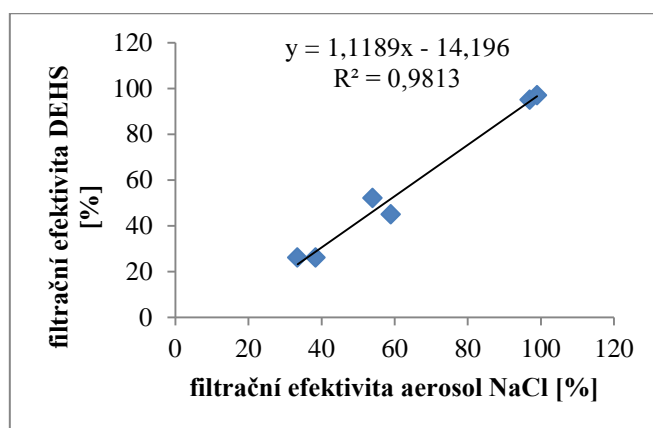
Obr. 23: Vztah efektivity záchytu pomocí aerosolu DEHS a aerosolu NaCl.
