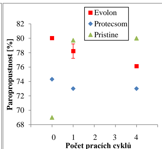
Obr. 31: Změna paropropustnosti textilí po údržbě
