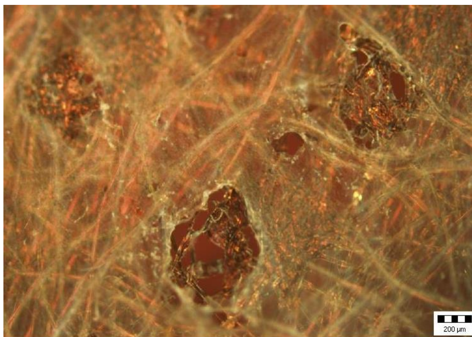
Materiál NW 40 prostřední vrstva rozlepení vrstev po vyprání
