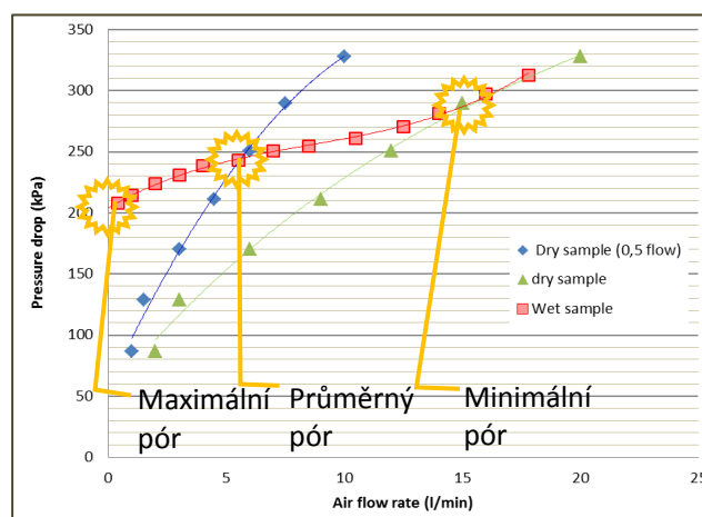
Obr. 25: Ukázka stanovení tlakového spádu pro výpočet velikosti póru [28]
