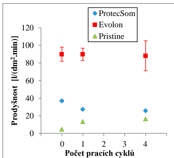
Obr. 30: Změna prodyšnosti textilí po údržbě
