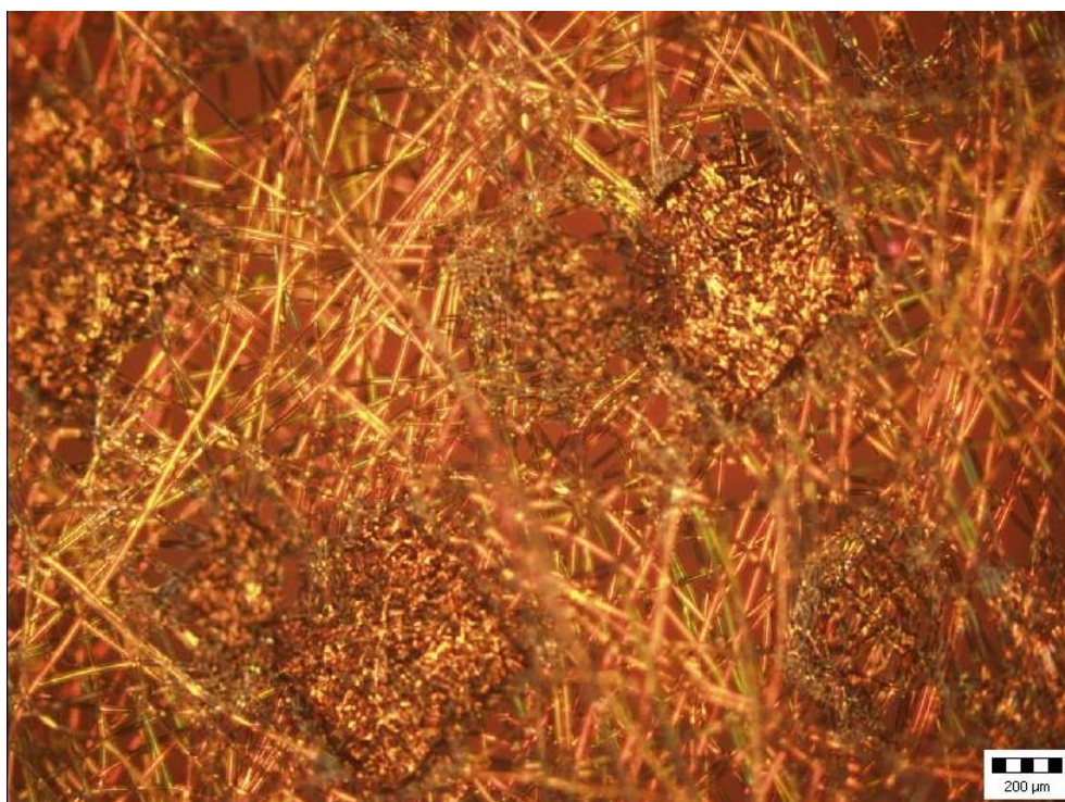
Materiál NW 40 rubní strana po rozlepení vrstev po vyprání
