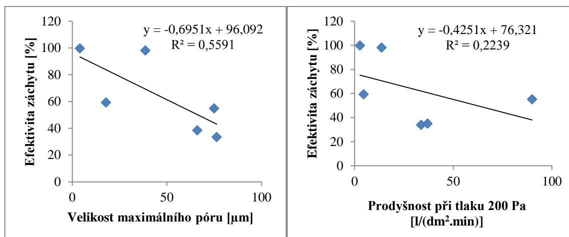
Obr. 28: Vztah efektivity záchytu a velikosti maximálního póru
