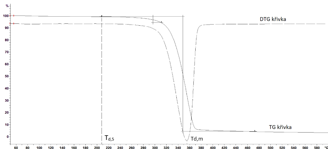
Obr. 3.10 Termogravimetrická křivka pro PLLA/KS
