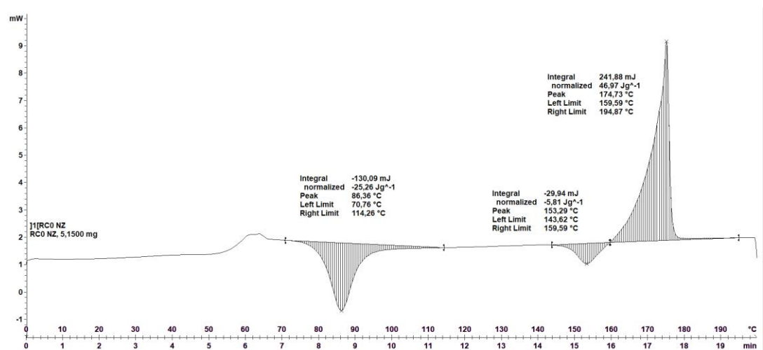
P2/1 Křivka diferenciální snímání kalorimetrie PLLA/KS při 0. recyklaci před stárnutím fáze prvního ohřevu
