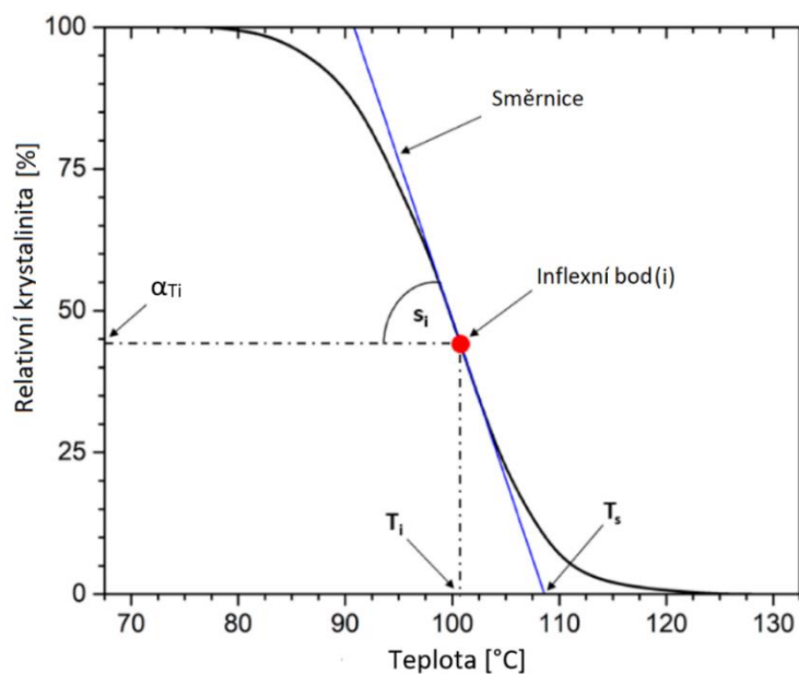
Obr. 3.24 Vyhodnocení neizoterní kinetiky krystalizace dle metody Kratochvíla a Kelnara
