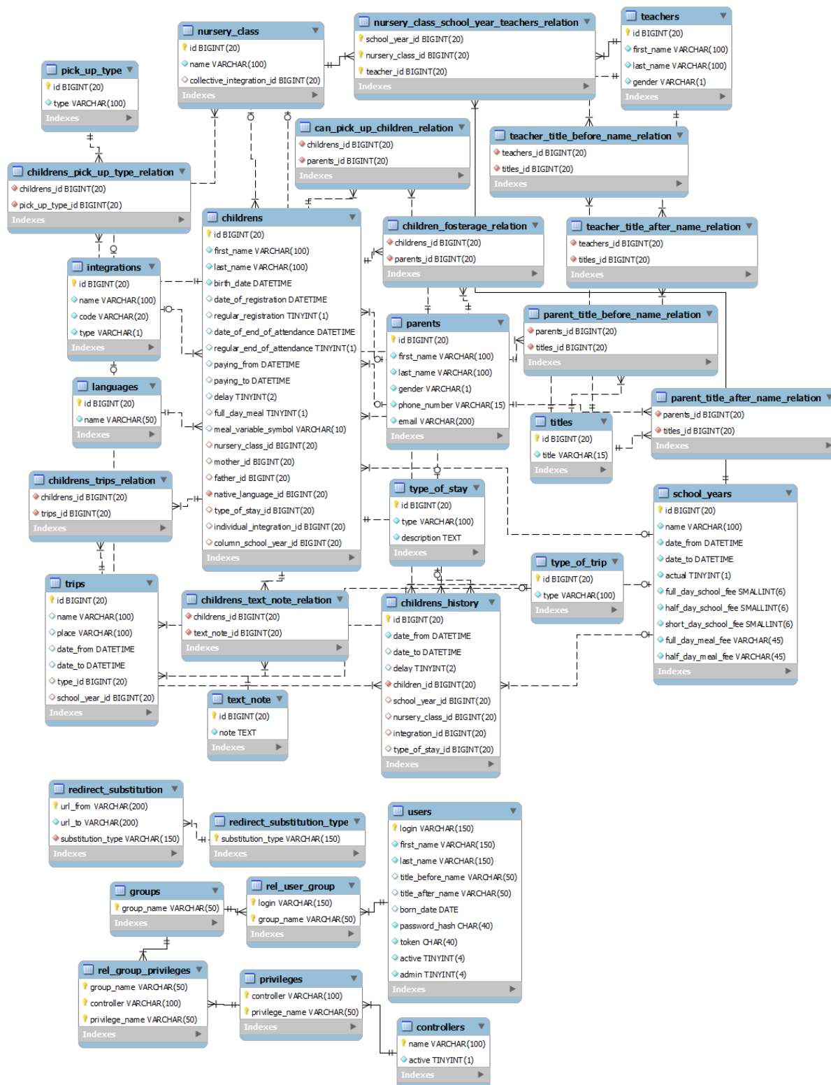
Obrázek 2 – struktura databáze
