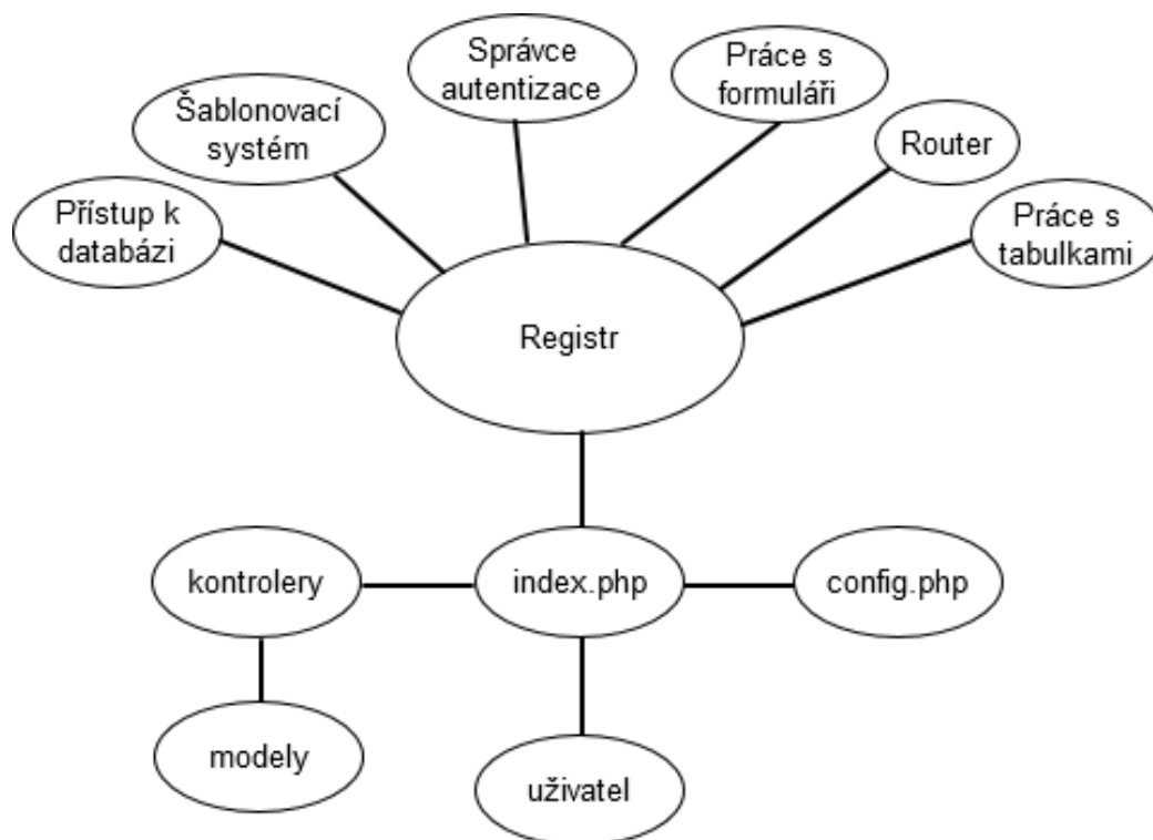
Obrázek 1 – struktura aplikace
